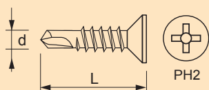
WKRETY SAMOWIERTNE DO STOLARKI PCV, bez wypustów, ocynkowane na biało SELF DRILLING WINDOW SCREWS, without ribs, white zinc plated
