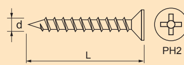
WKRETY DO MONTAŻU OKUĆ łeb stożkowy płaski, bez wypustów, ocynkowane na biało SELF TAPPING SCREWS FOR WINDOW FITTINGS, flat head, without ribs, white zinc plated
