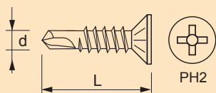
WKRETY SAMOWIERTNE DO STOLARKI PCV, z wypustkami, ocynkowane na biało SELF DRILLING WINDOW SCREWS, with ribs, white zinc plated
